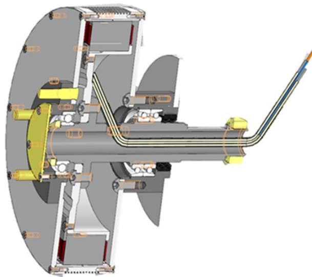
Рис. 3. Разрез мотора. 3D-модель автора
