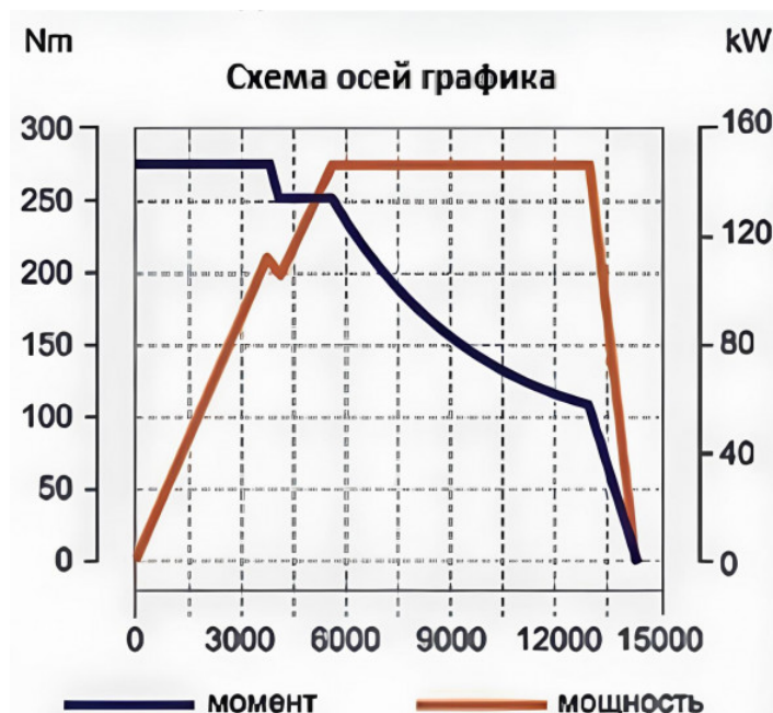
Рис. 2. Графики изменения крутящего момента и мощности электродвигателя 8
