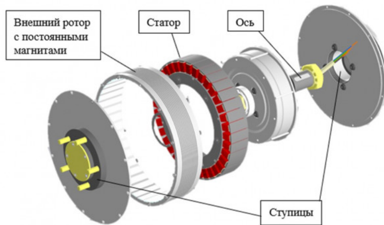
Рис. 4. Сборочные единицы и детали мотора [Тишкевич: 361]
