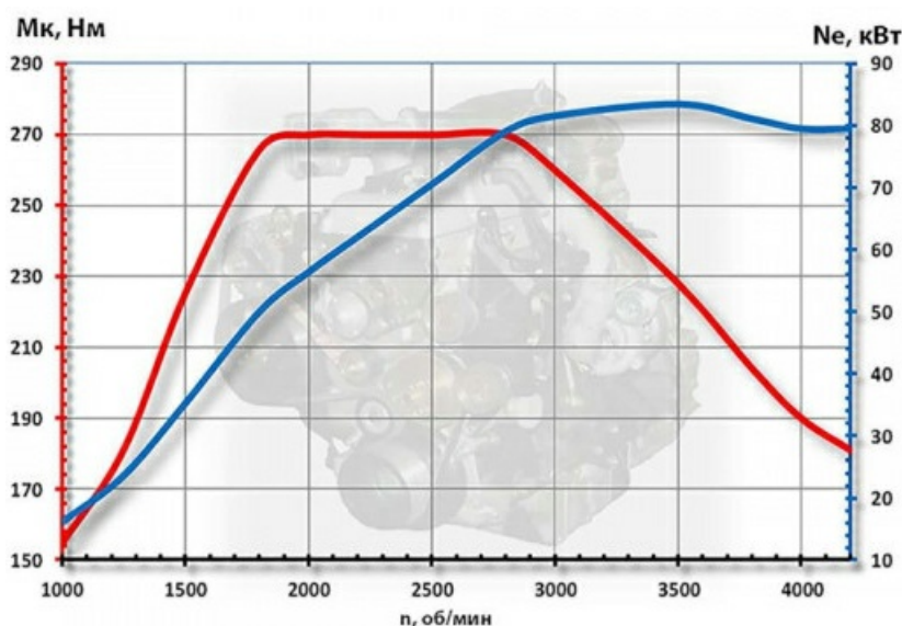
Рис. 1. Графики изменения крутящего момента и мощности ДВС 2
